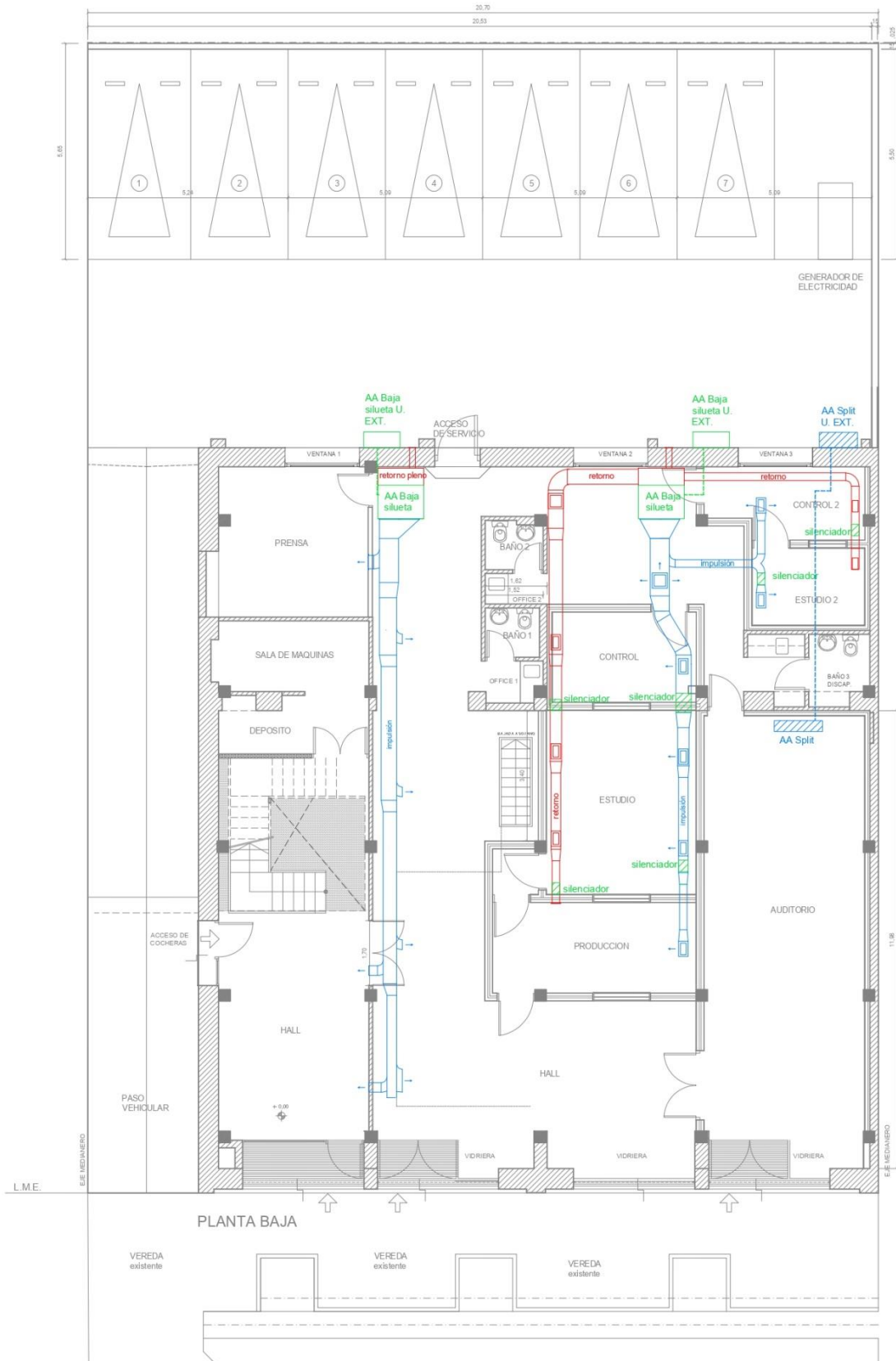
PLANTA BAJA escala 1:50
